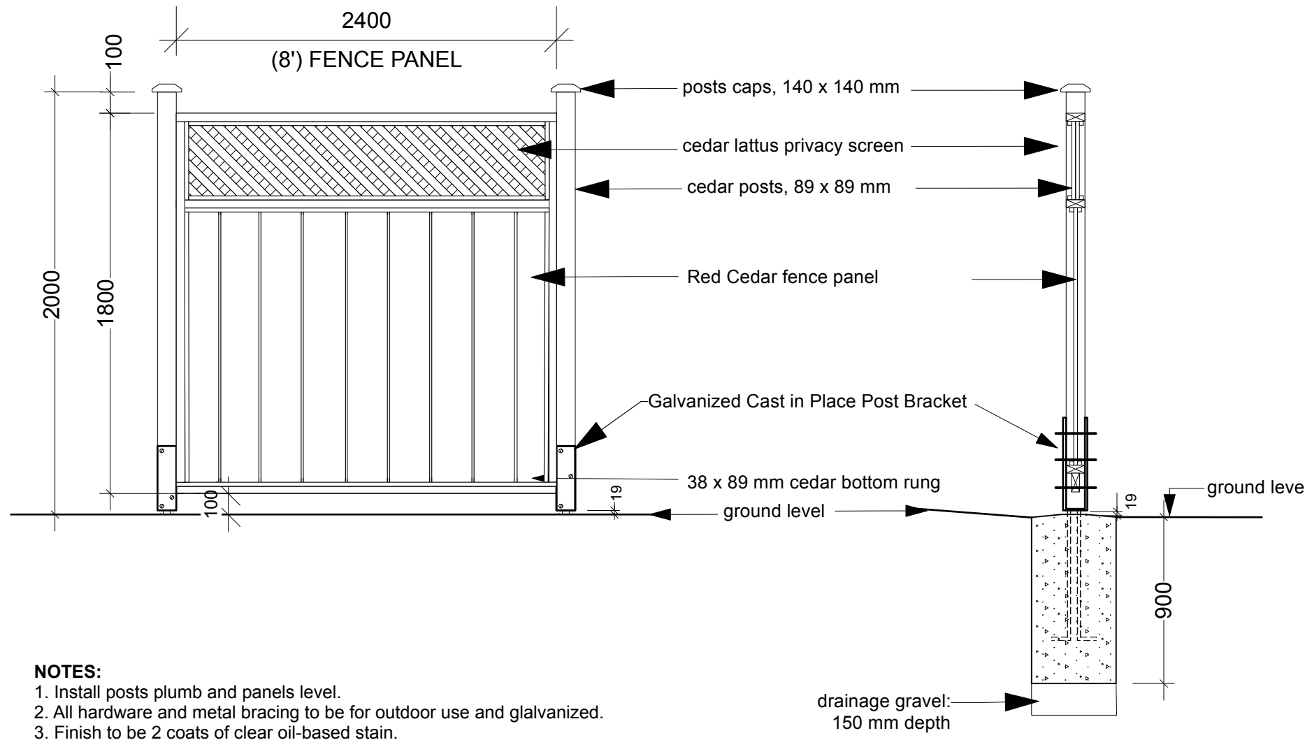
1 Cedar Fence - Elevation & Section L-3 Scale: 1:25
